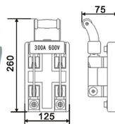
尺寸圖 DIMENSION
