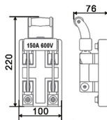
尺寸圖 DIMENSION
