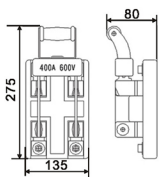
尺寸圖 DIMENSION
