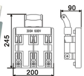
尺寸圖 DIMENSION
