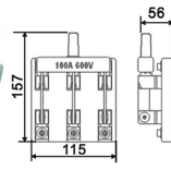
尺寸圖 DIMENSION
