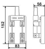
尺寸圖 DIMENSION
