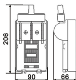
尺寸圖 DIMENSION
