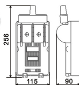
尺寸圖 DIMENSION
