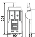
尺寸圖 DIMENSION
