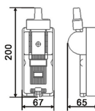
尺寸圖 DIMENSION
