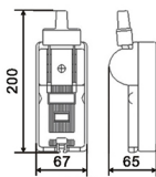
尺寸圖 DIMENSION
