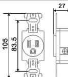
尺寸圖 DIMENSION
