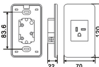
尺寸圖 DIMENSION
