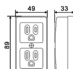
尺寸圖 DIMENSION
