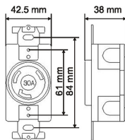
尺寸圖 DIMENSION
