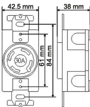
尺寸圖 DIMENSION
