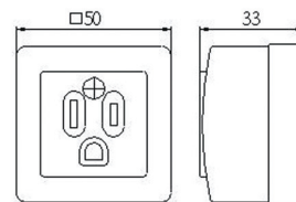
尺寸圖 Dimension
