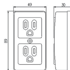
尺寸圖 Dimension
