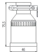
尺寸圖 Dimension
