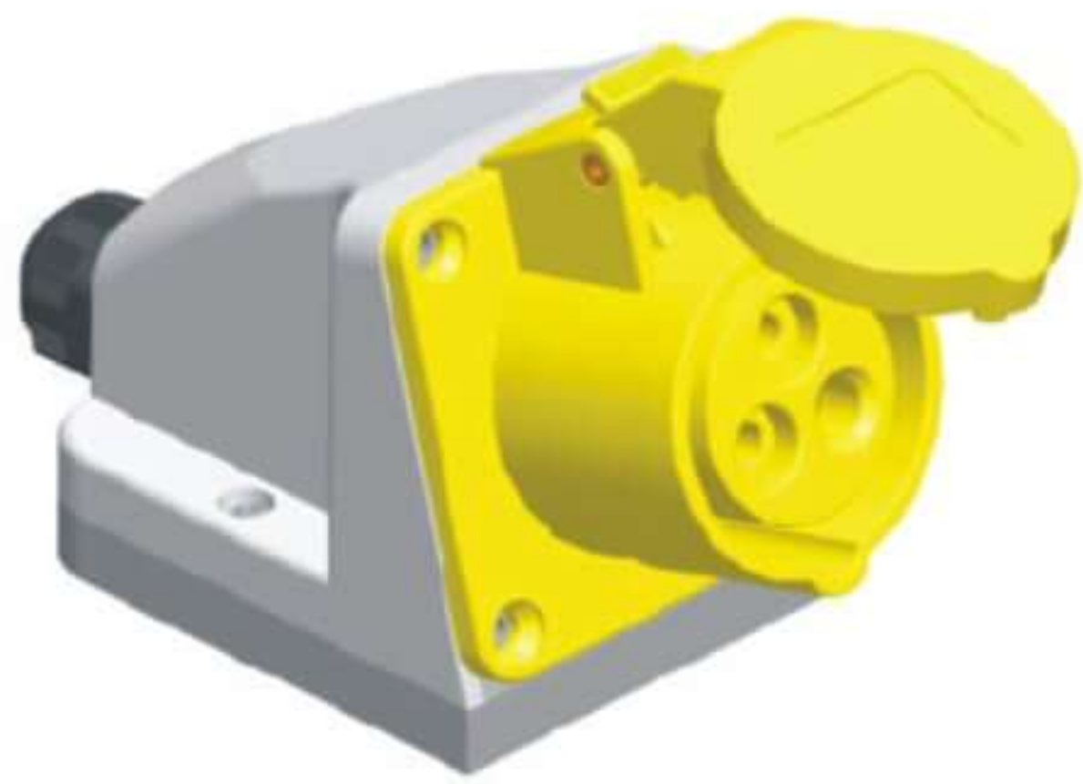
》 SFC-S324-3-BOX (16A/130V) 》 SFC-S324D-2-BOX (32A/130V) 2P+E
